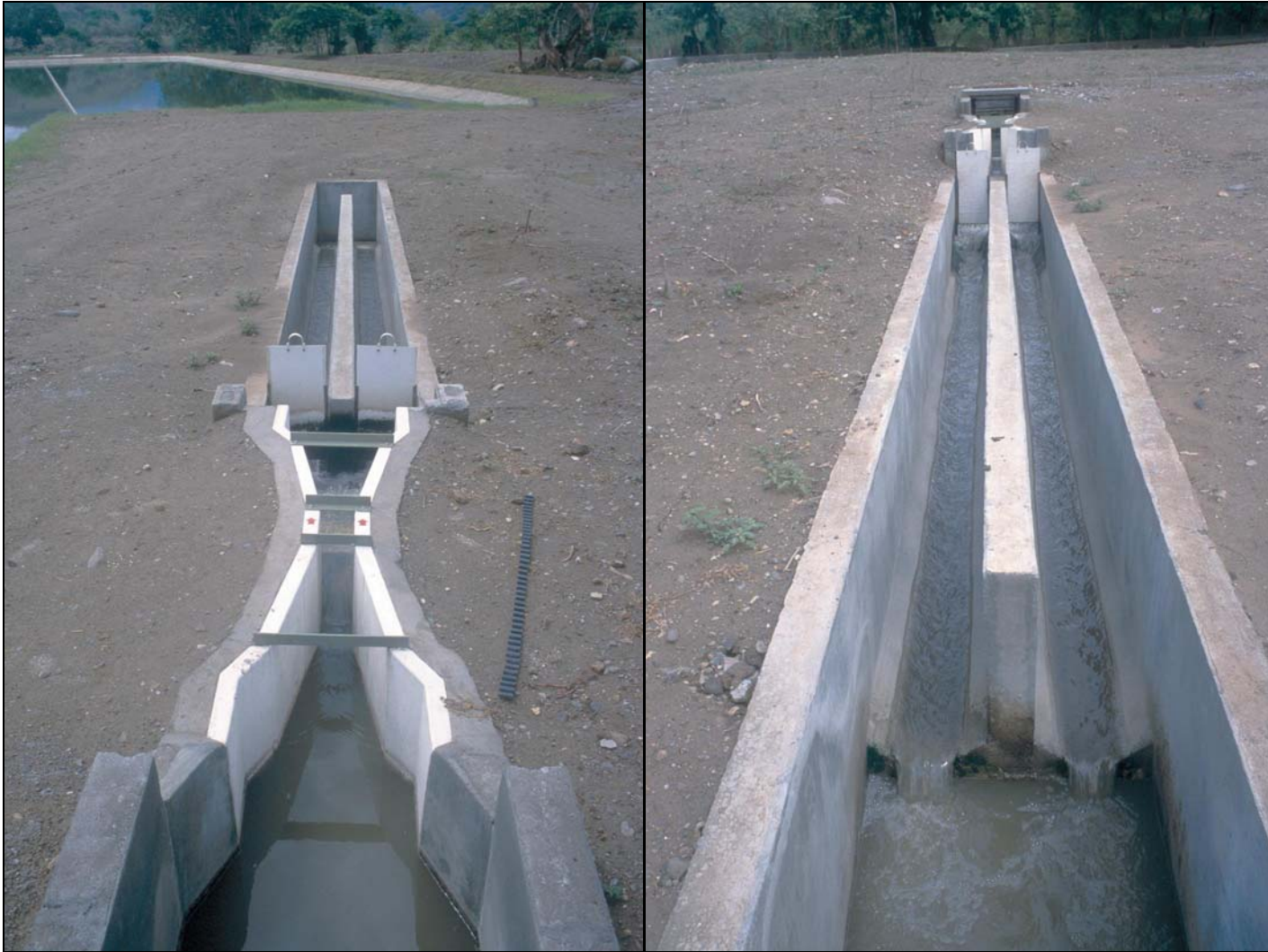
Fotos 6-7: Este desarenador fue construido sin drenaje y, además, sin vertederos en la salida para controlar la velocidad horizontal. La canaleta Parshall prefabricado, lo que no se puede utilizar para medir caudales porque el contratista cortó el fondo para instalarla, debería de haber ubicada después del desarenador como se discutió en detalle en el Capítulo 3; en este caso no necesitarían vertederos adicionales. Este caso es típico de problemas encontrados con diseño y supervisión de construcción. (Trinidad, Honduras)
