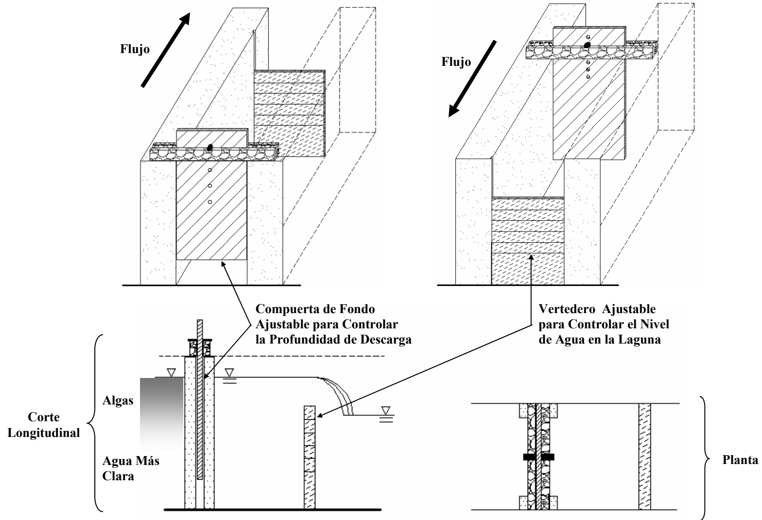
Figura 6-4: Los detalles del diseño físico de i) una compuerta de fondo ajustable para optimizar la calidad del efluente en términos de sólidos suspendidos causados por la banda de algas en la laguna; y ii) un vertedero rectangular ajustable para controlar el nivel de agua en la laguna. El vertedero ajustable utiliza una serie de compuertas de altura corta.
