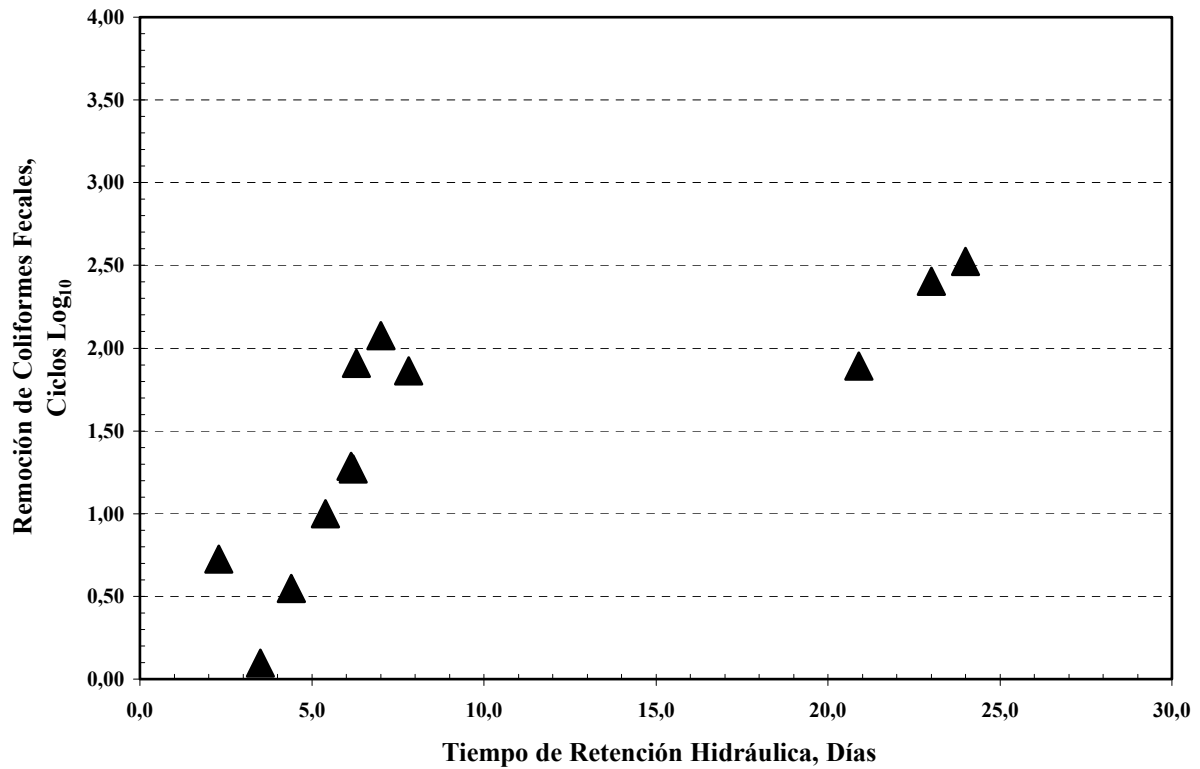
Figura 2-3: Remoción de Coliformes Fecales en Lagunas Primarias
