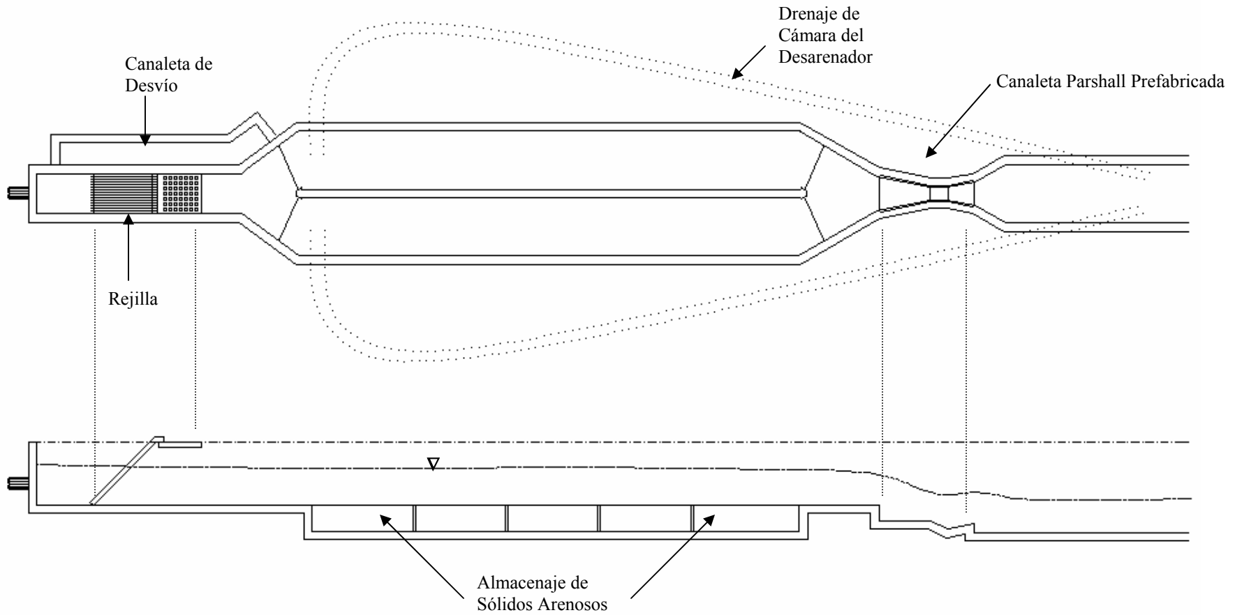
Figura 3-1: La Instalación Recomendada de Rejilla, Desarenador Horizontal con Dos Cámaras, y Canaleta Parshall para el Control de Velocidad y Medición de Caudal.
