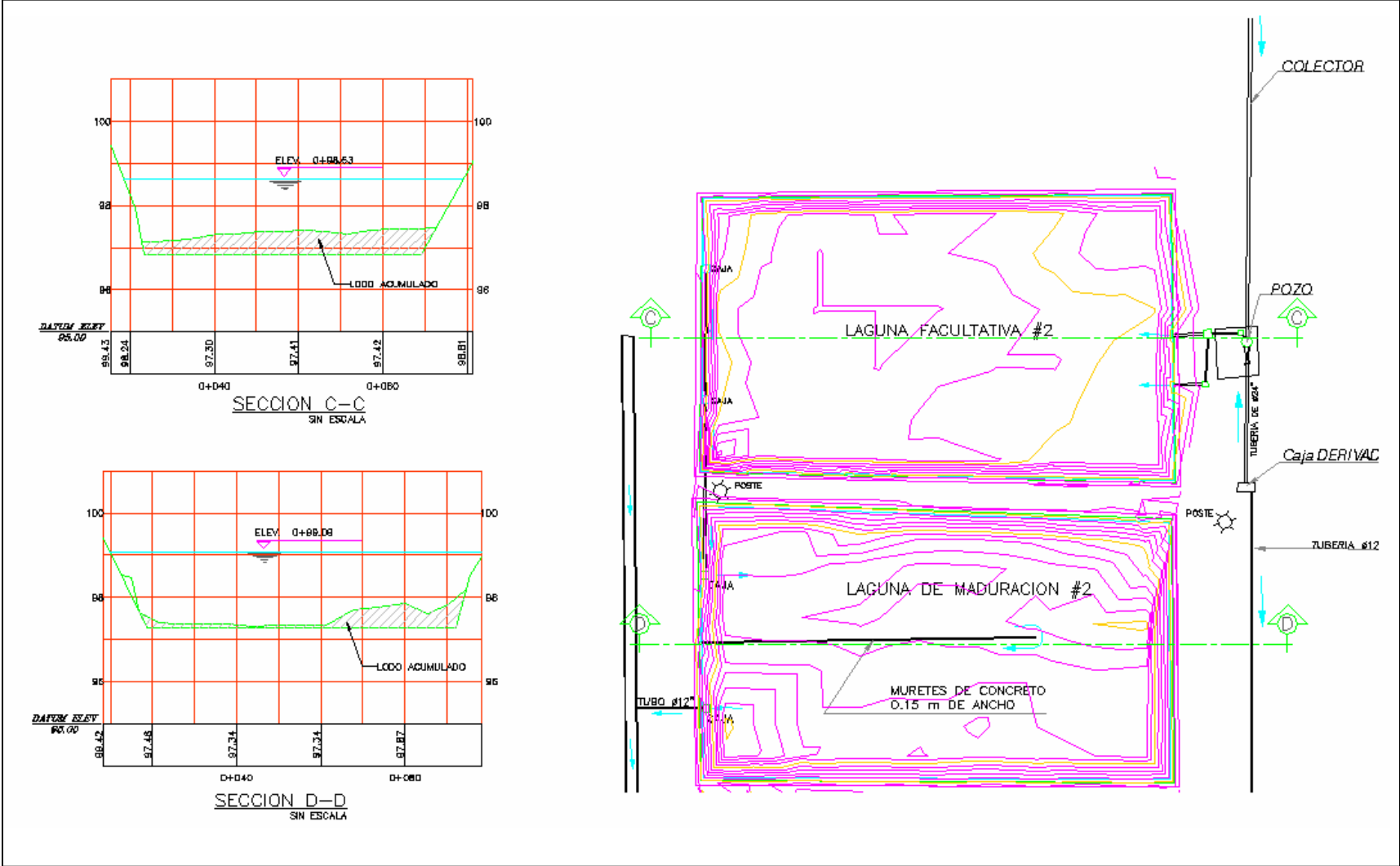
Figura 8-4: Resultados del Estudio de Batimetría de la Laguna Facultativa II, Villanueva, Cortés
