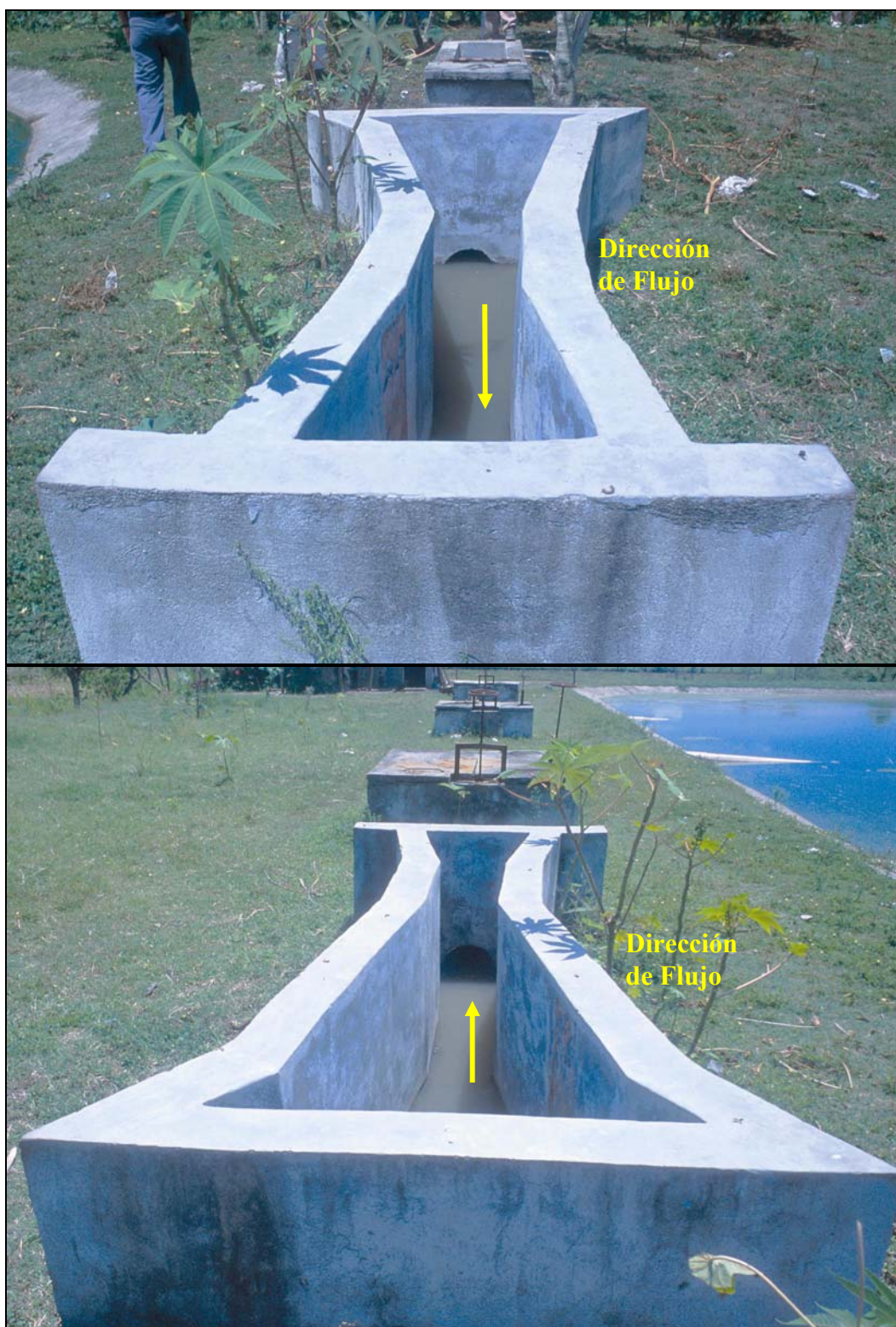
Fotos 3-13: Otro ejemplo de la mala construcción de una canaleta Parshall de concreto que también no tiene flujo libre por el mal diseño del pendiente. (Choloma, Honduras)
