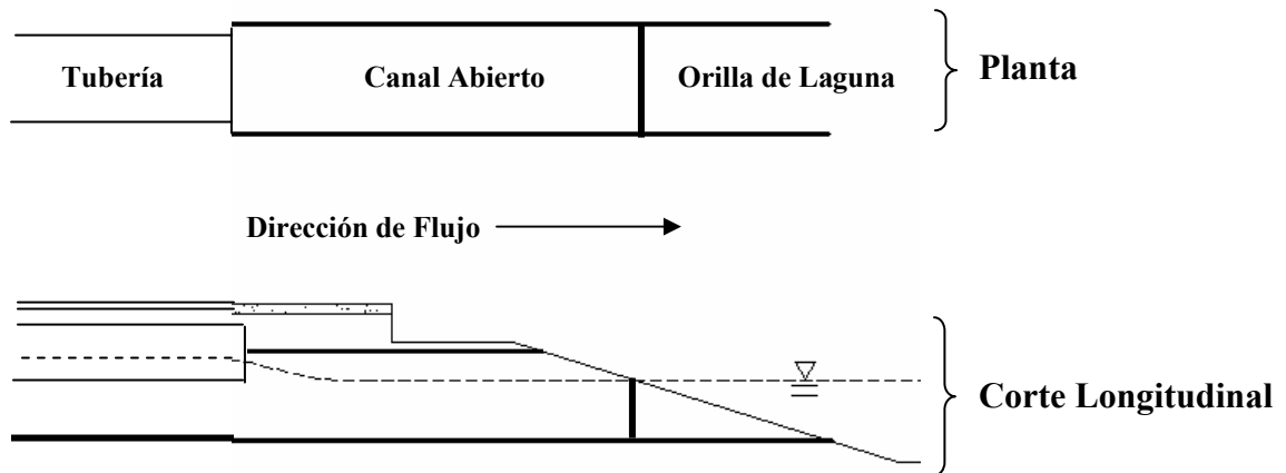
Figura 6-1: Las entradas en todas las lagunas deben ser de canales abiertos que descargan al nivel de agua, lo que promueve flujo de tipo pistón por el choque entre el caudal entrante y la masa de agua en la laguna.
