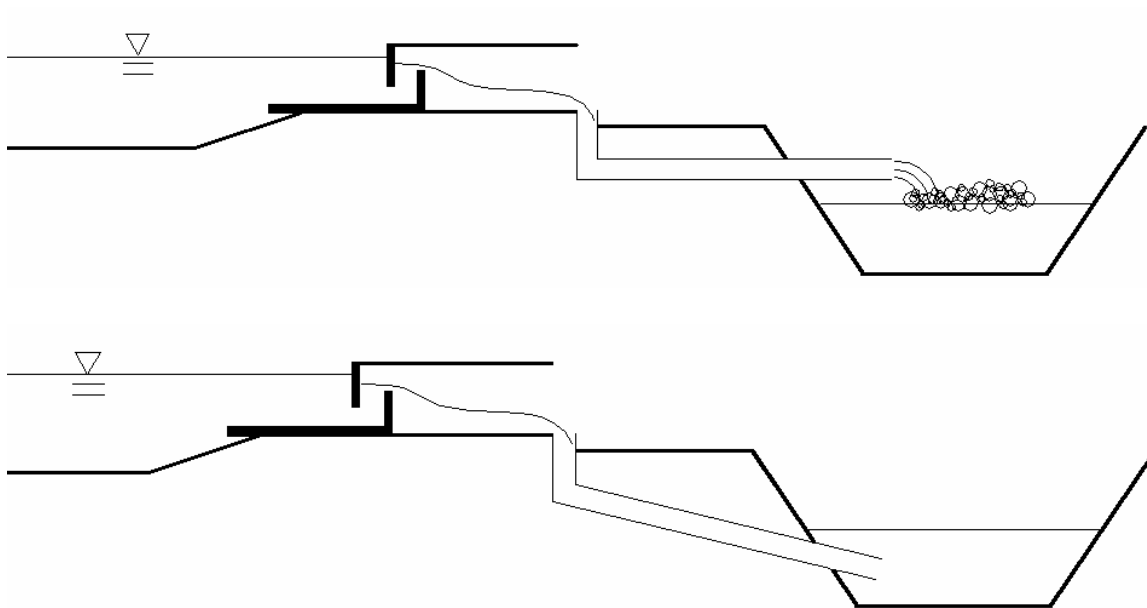
Figura 6-5: Un problema con la descarga del efluente final arriba del nivel de agua en el cuerpo receptor es la producción de espuma causada por detergentes y otros tensoactivos no biodegradables en las aguas residuales (Véase las Fotos 6-15). La manera más eficaz controlar la espuma es el uso de dispositivos de descarga final abajo el nivel de agua en el cuerpo receptor.
