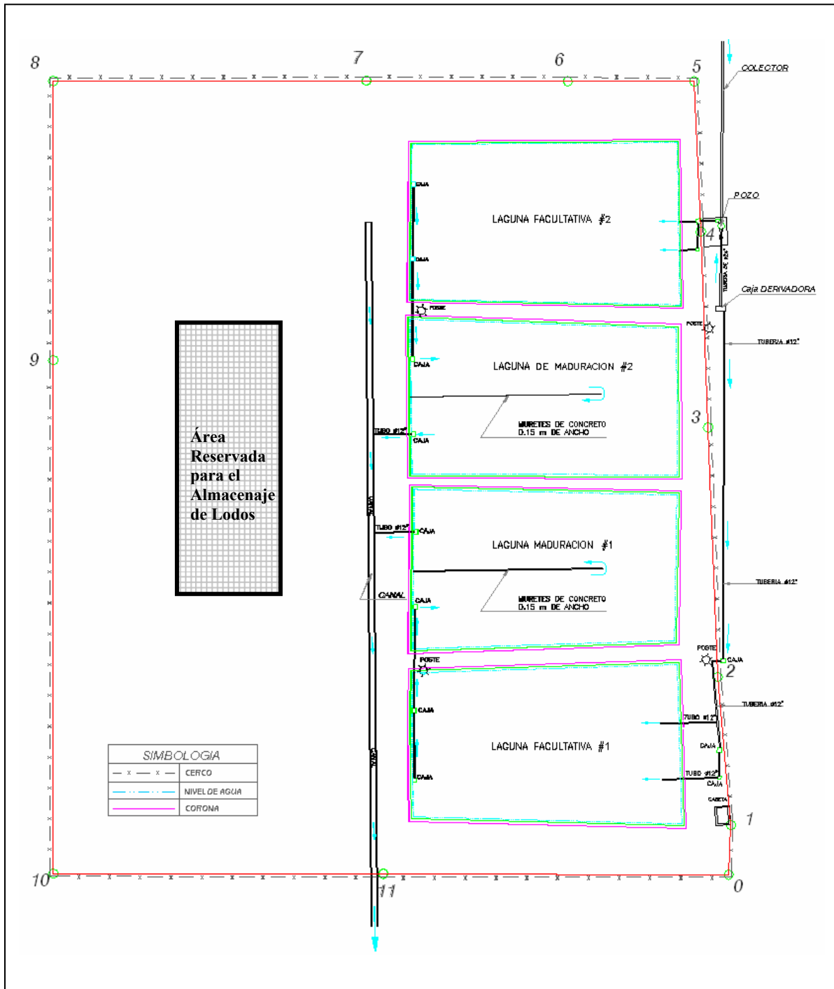
Figura 8-2: Instalación de las Lagunas de Estabilización de Villanueva, Cortés
