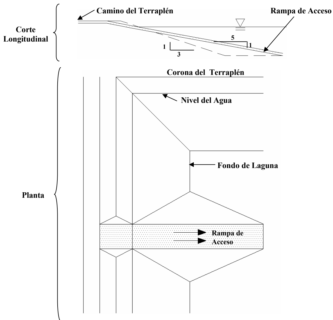
Figura 6-7: Cada laguna primaria debe incluir rampas de acceso hasta al fondo para maquinaria como cargadores frontales y volquetes para permitir la remoción de lodos. Las rampas tienen que ser pavimentadas para que la maquinaria tenga tracción sin dañar la impermeabilización y taludes de la laguna.
