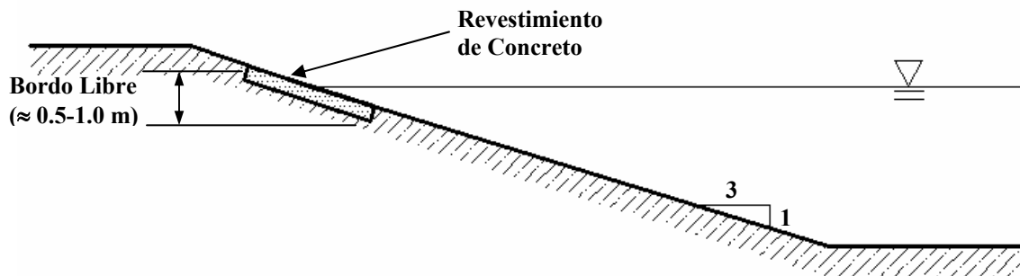
Figura 6-6: El diseño del talud interior debe incluir un revestimiento de concreto en la orilla para evitar el crecimiento de plantas acuáticas y erosión por la acción de olas. El borde libre del revestimiento debe cubrir los niveles de agua encontradas en la operación durante la época seca y lluviosa. Típicamente el talud interior tiene una relación de 3/1 (horizontal/vertical).
