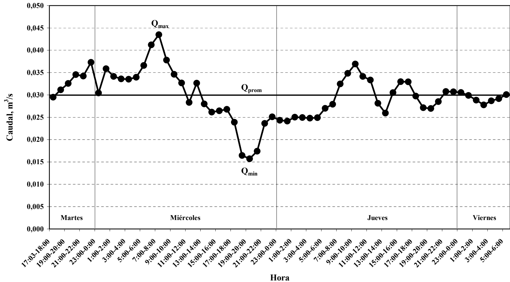
Figura 3-7: Medición de Caudales en Sistema de Lagunas de Catacamas Sector Este (02-05/09/03)
