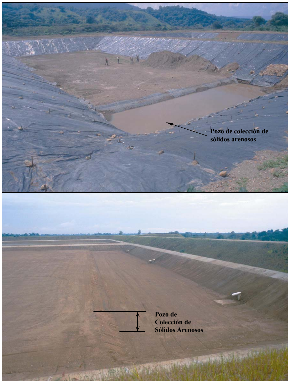
Fotos 3-14: Ejemplos de pozos de colección de sólidos arenosos instalados en la entrada de la laguna primaria en vez de utilizar un desarenador. La foto arriba (Boca del Monte, Guatemala) es una laguna anaeróbica y abajo (El Paraíso, Honduras) una facultativa. Esta práctica no es recomendable por la dificultad de remover los lodos cuando sea necesario (Véase el Capítulo 8).
