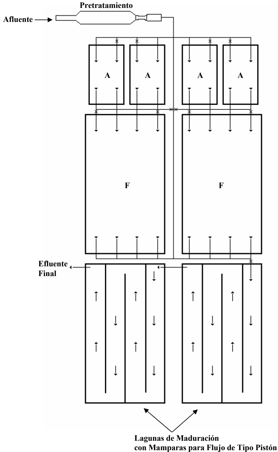
Figura 4-3: Dos baterías en paralelo de dos lagunas anaeróbicas y una facultativa, seguidas por dos lagunas de maduración en serie. Se utiliza lagunas en paralelo para poder tener una fuera de servicio para la remoción de lodos. Las lagunas anaeróbicas disminuyen el área total del sistema, pero requieren mucho mantenimiento y generalmente no se recomienda su uso en las municipalidades.
