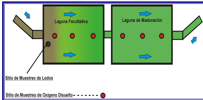
Figura 2-2: Esquemas Mostrando la Ubicación de Puntos de Muestreo Dentro Lagunas
