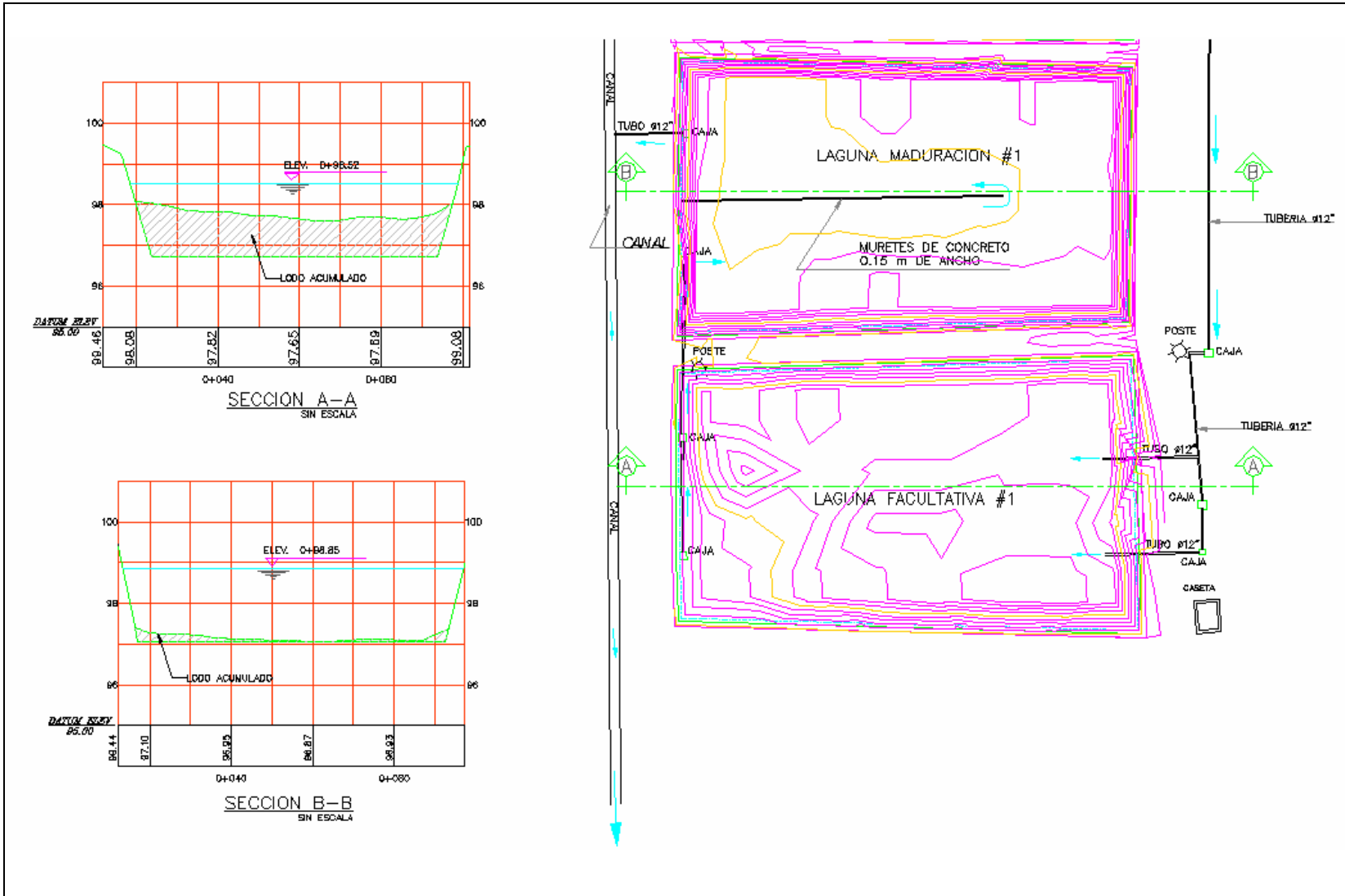
Figura 8-3: Resultados del Estudio de Batimetría de la Laguna Facultativa I, Villanueva, Cortés
