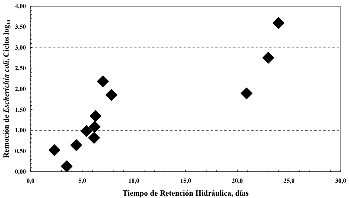
Figura 2-4: Remoción de Escherichia coli en Lagunas Primarias
