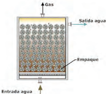
Filtro anaerobio
