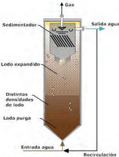
Reactor anaerobio de lecho expandido (EGSB) *Sistema de transición entre la segunda y tercera generación.
